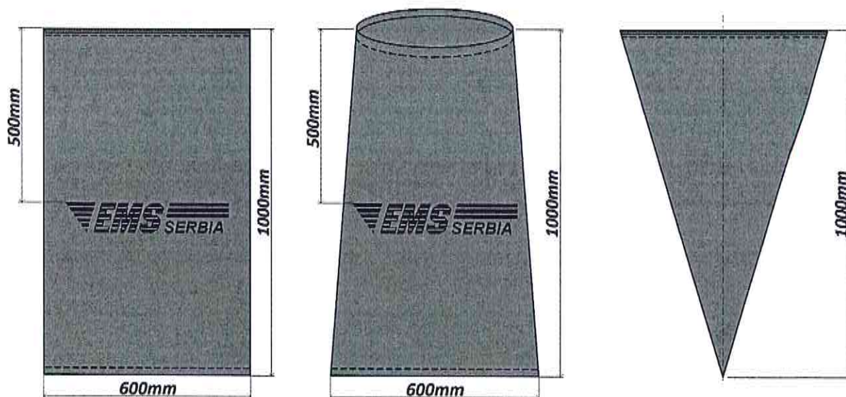
Цртеж бр. 1 - Изглед и димензије вреће EMS полипропилен наранџаста 600x1000mm
