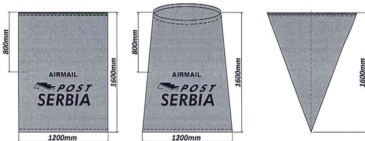
Цртеж бр. 5 - Изглед и димензије вреће за авионске пакетске пошिल्ке полиестер плава 1200×1600mm
