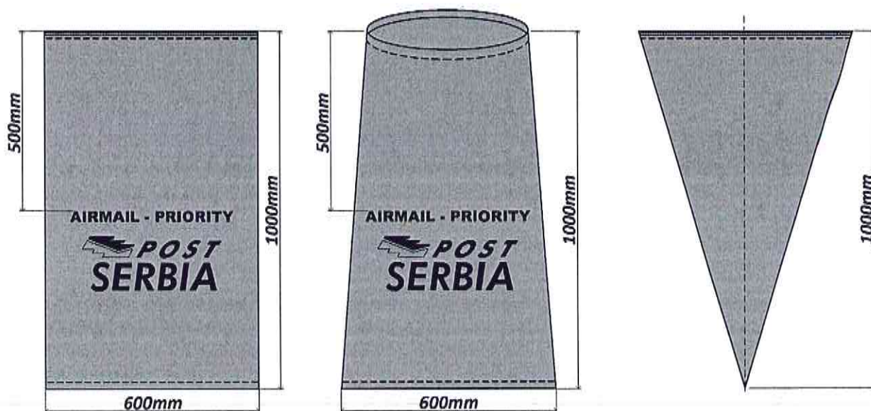
Цртеж бр. 3 - Изглед и димензије вреће за авионске писмоносне поштоматке полипропилен плава 600×1000mm
