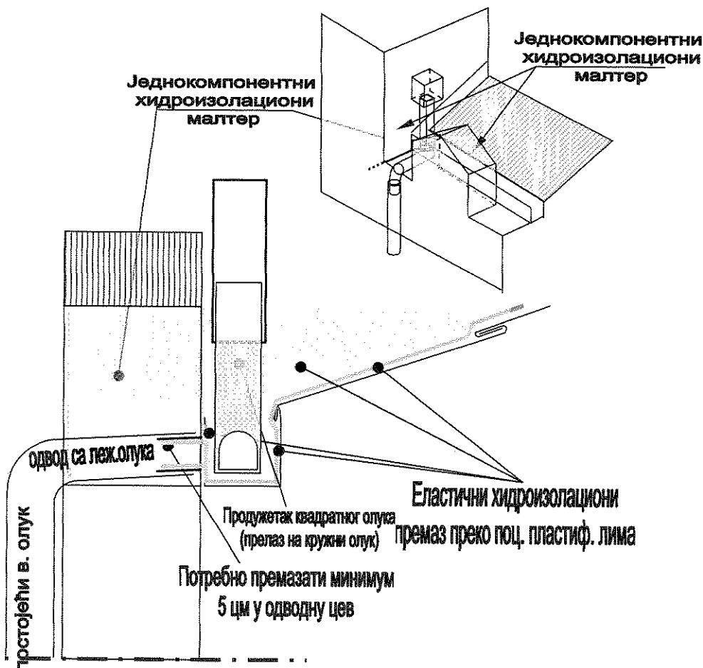
ЦРТЕЖ 11 (објекат Палмотићева 2)
