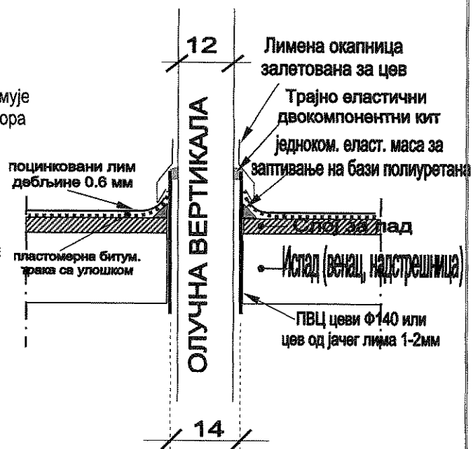
ЦРТЕЖ 2 (објект Палмотићева 2)
