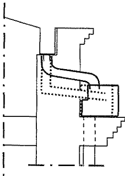
Промена облика лименог казанчића због несметаног функционисања постојеће вентилације (објекат Косовска 47)
