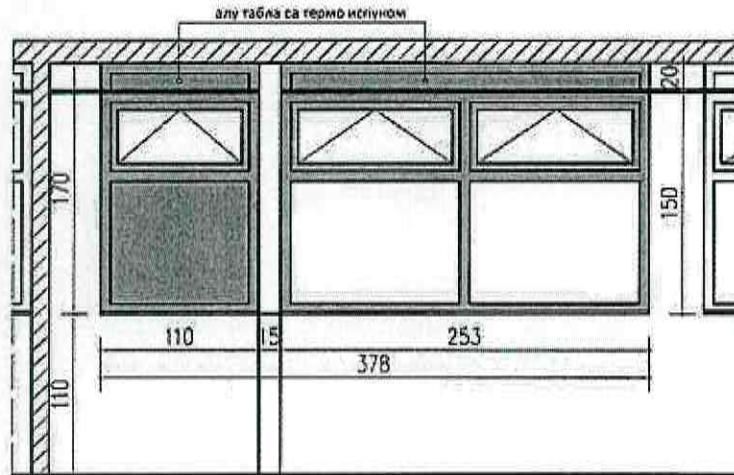
ИЗГЛЕД - ТРОКРИЛНИ ПРОЗОР R=1:50
