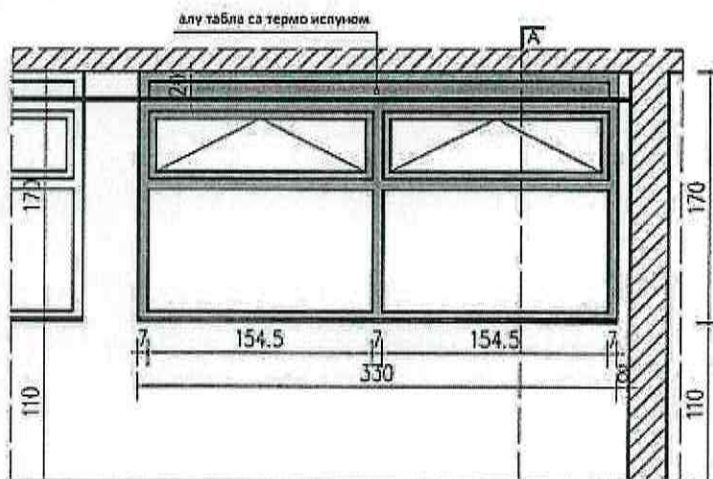
ИЗГЛЕД - ДВОКРИЛНИ ПРОЗОР R=1:50
