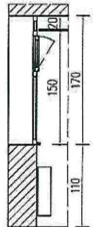
ПРЕСЕК А-А R=1:50
