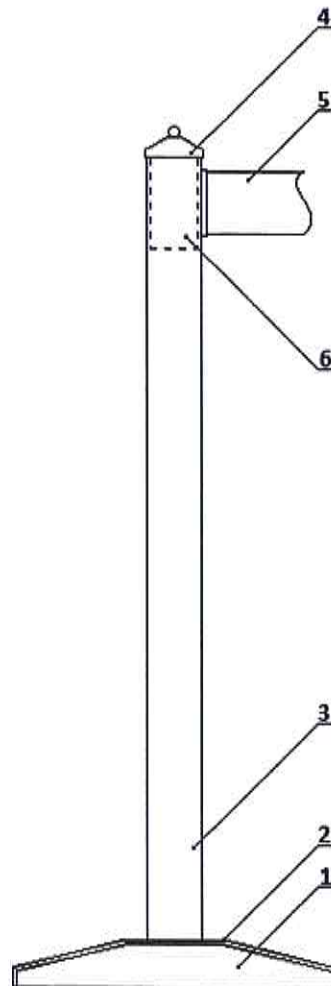
Цртеж бр.1 - Делови стубића за обележавање јединственог реда чекања
