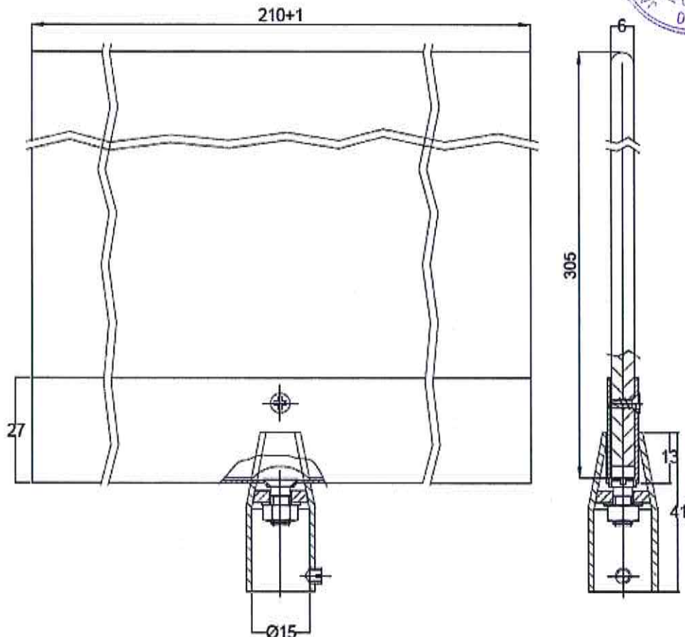
Цртеж бр.3 – Делови и димензије држача рекламног холдера
