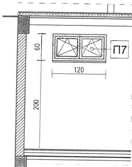
ИЗГЛЕД - ФАСАДНИ ПРОЗОР R=1:50
