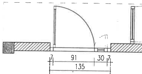
ОСНОВА - УНУТРАШЊИХ ВРАТА R=1:50
