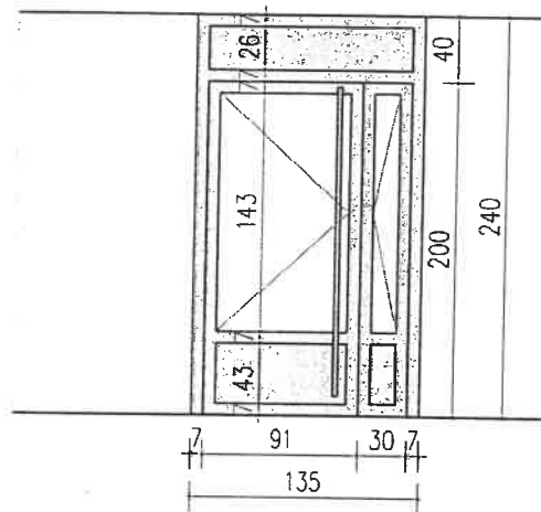
ИЗГЛЕД - УНУТРАШЊИХ ВРАТА R=1:50
