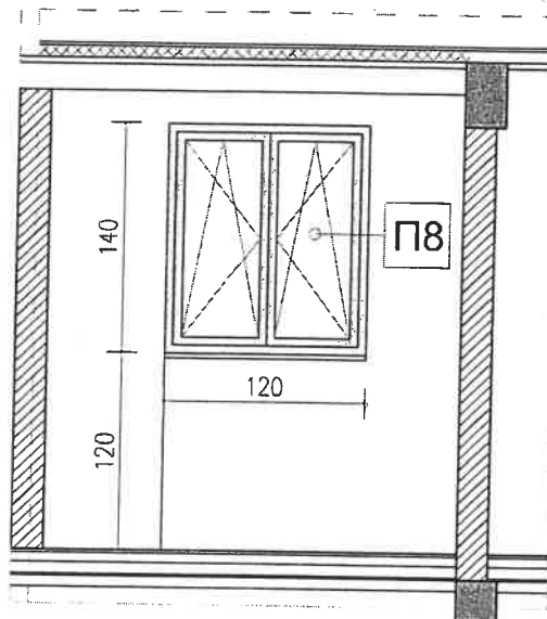
ИЗГЛЕД - ФАСАДНИ ПРОЗОР R=1:50
