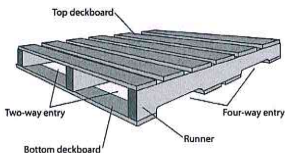
Слика 1. Палета стандардних ЕУРО димензија
