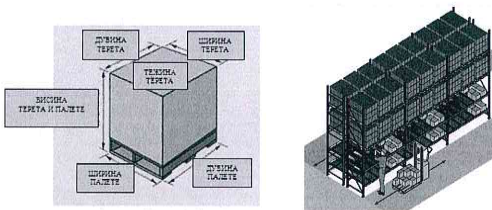
Слика 2. Складиштење палета у регале
